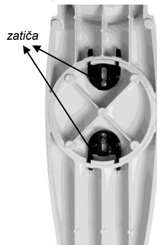
Slika 3: Spodnji del rezalnika od zadaj.
